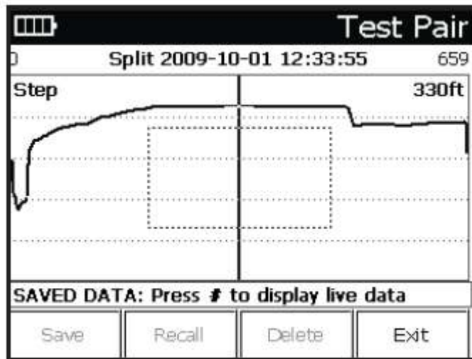
Разбиение пары
