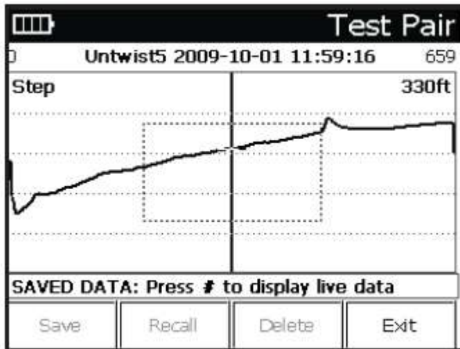
Нескрученная пара
